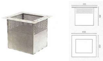
7. caisson d’oxygénation - Clarova TLV 2333
