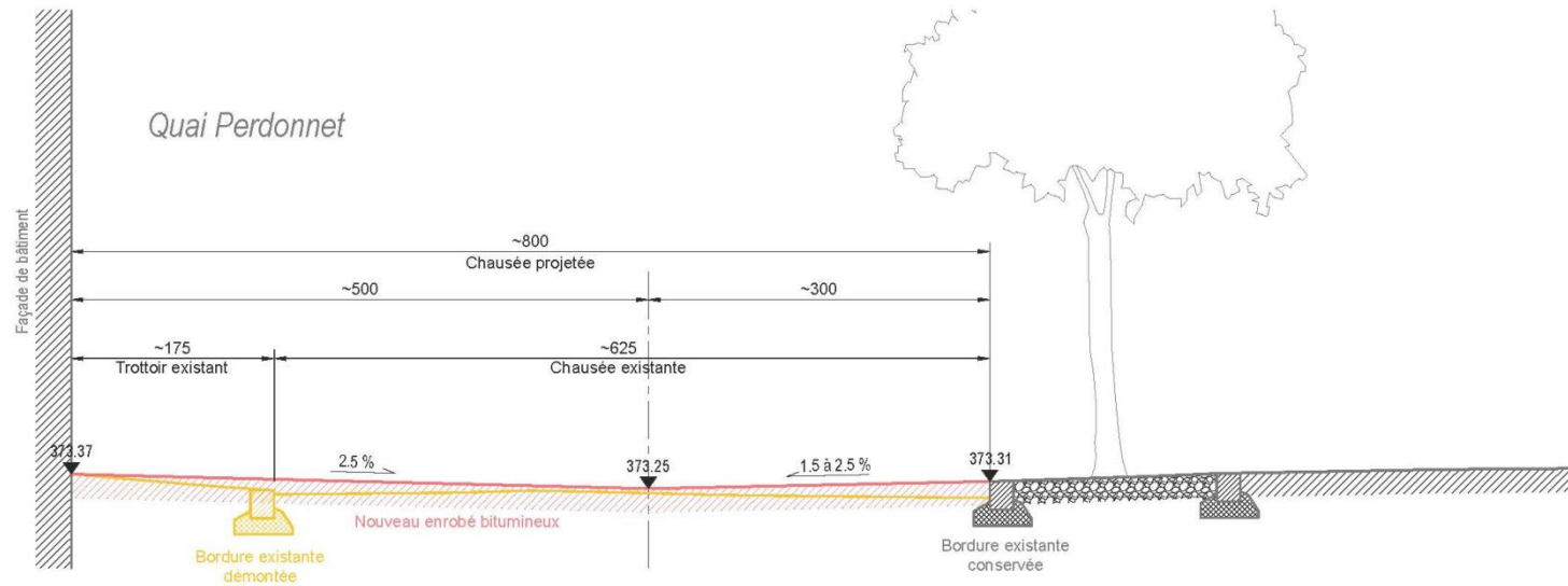
Profil en travers type
